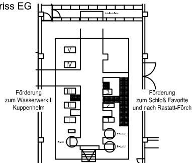
Grundriss EG
